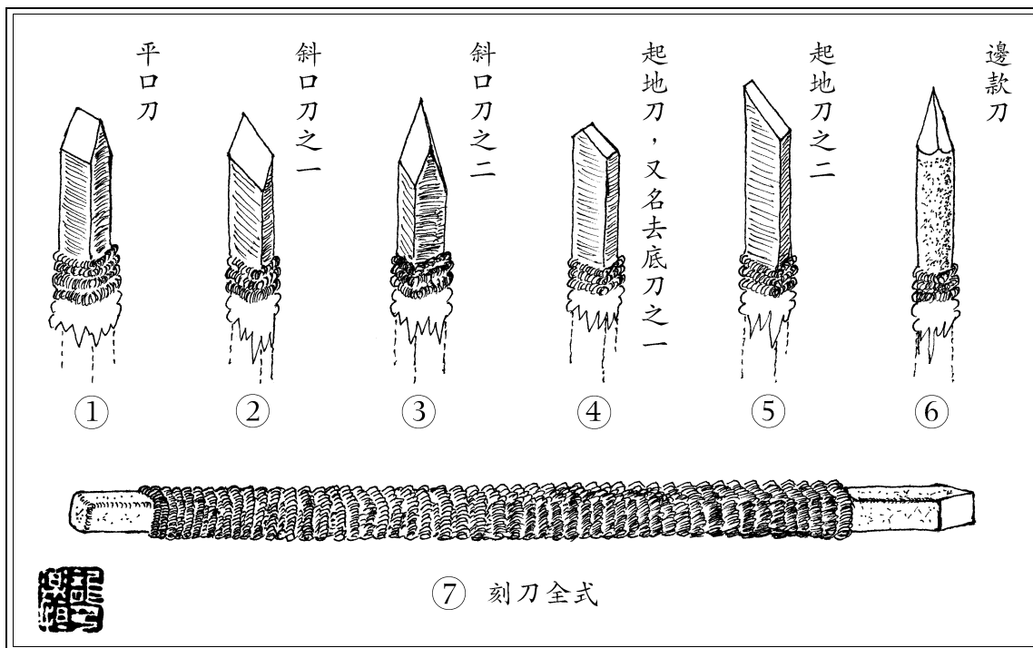
fig. 1: les différents couteaux à graver les sceaux 篆刻刀式
